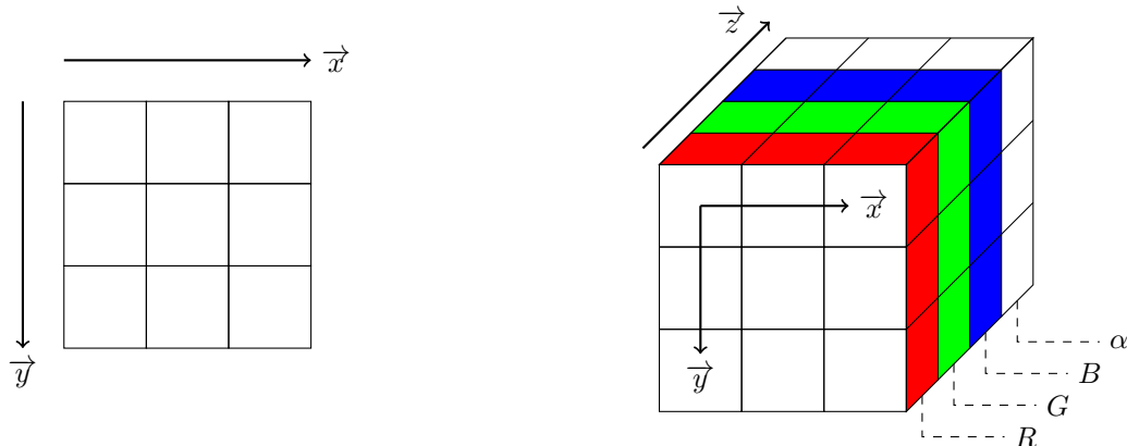
FIGURE 1 – Principe de stockage des images en niveaux de gris (gauche) et en couleur (droite).
